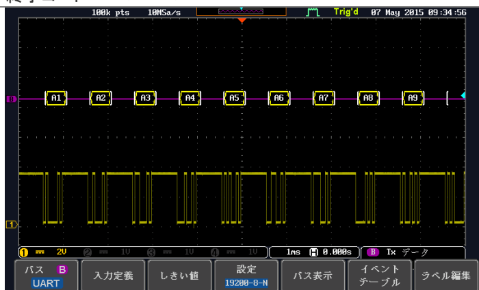
UART 表示例
