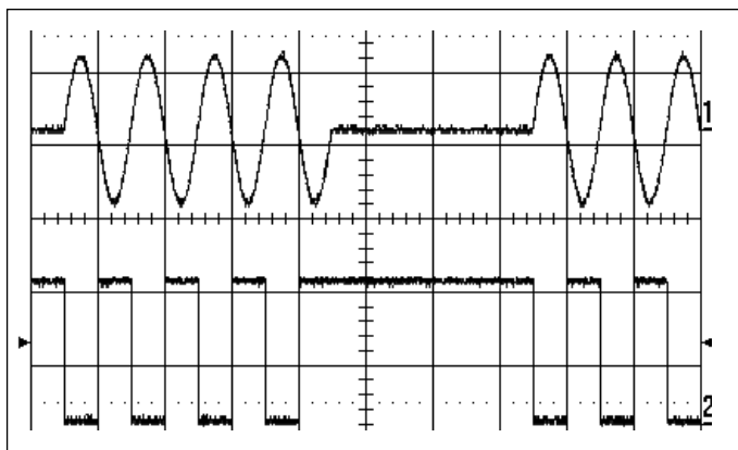
正弦波のバースト波形
