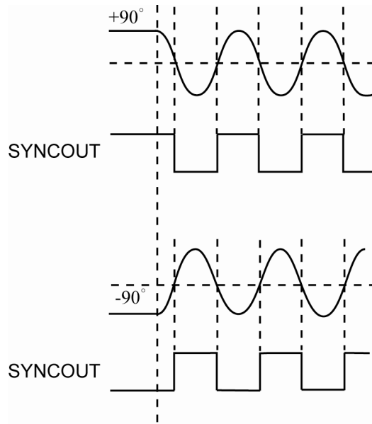
初期位相を \pm 90^\circ にした場合の正弦波
