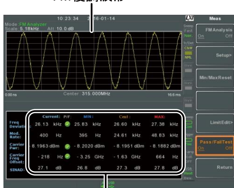
FM変調の測定値
