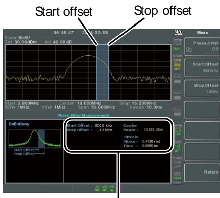
位相ジッタ測定
