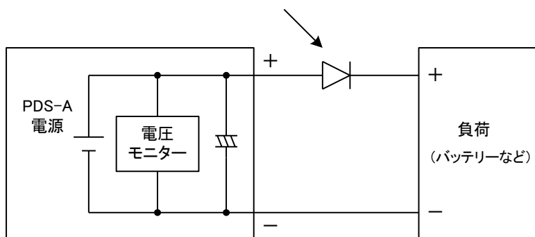
図 4-1 エネルギーを持った負荷の接続
