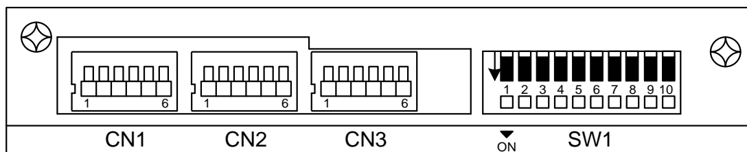
図 9-1 標準ボードのコネクタとディップスイッチ
