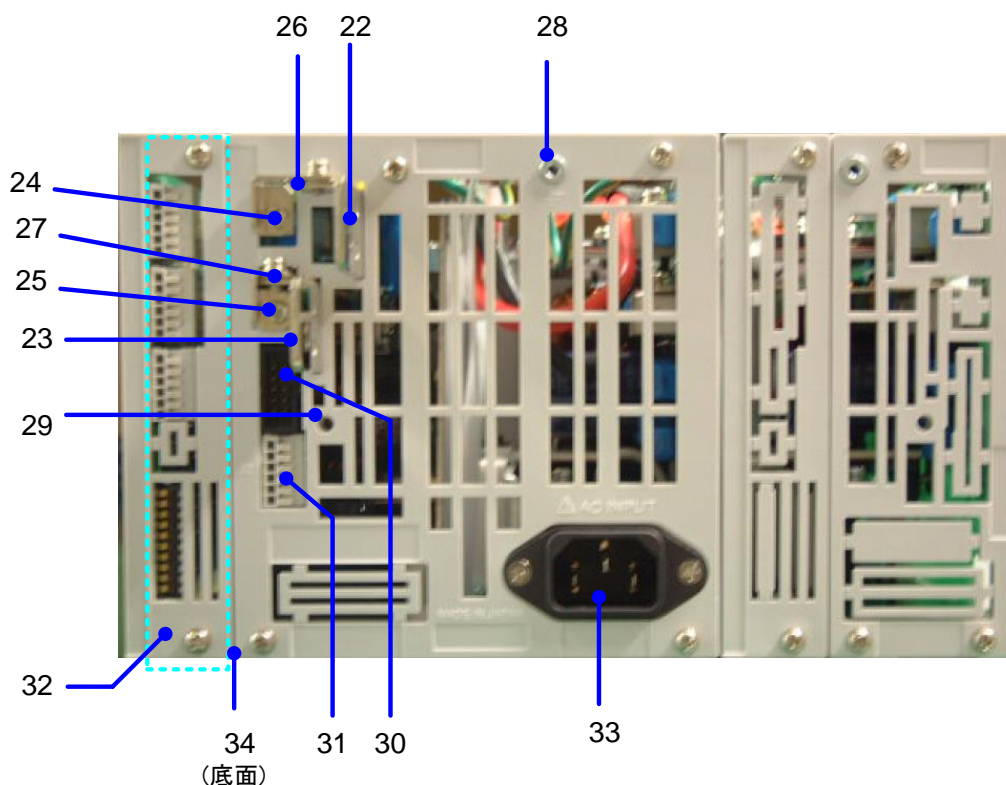
図 3-3 背面パネル
