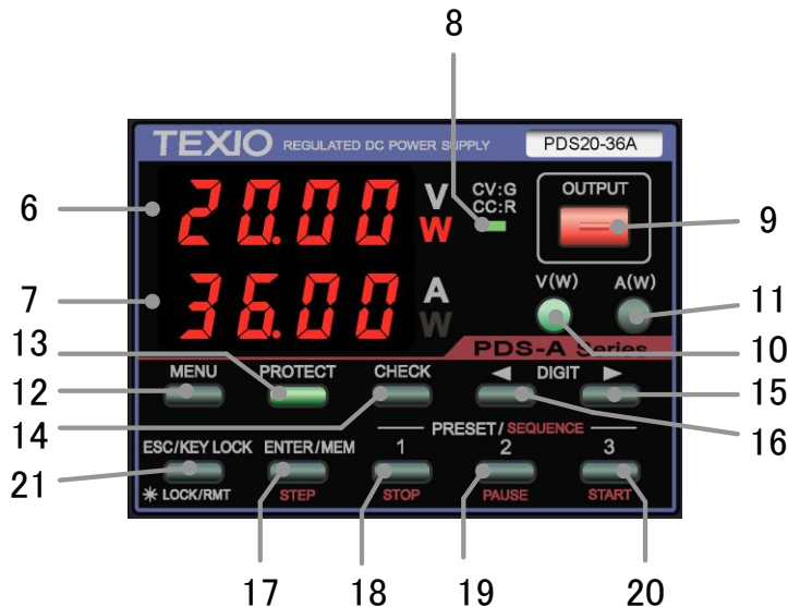
図 3-2 操作パネル部
