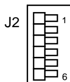
図 3-4. J2 コネクタのピン番号
