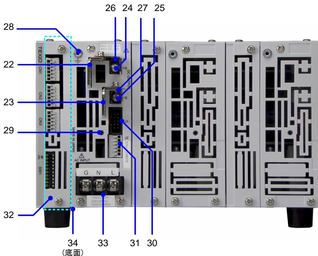
図 3-3 背面パネル
