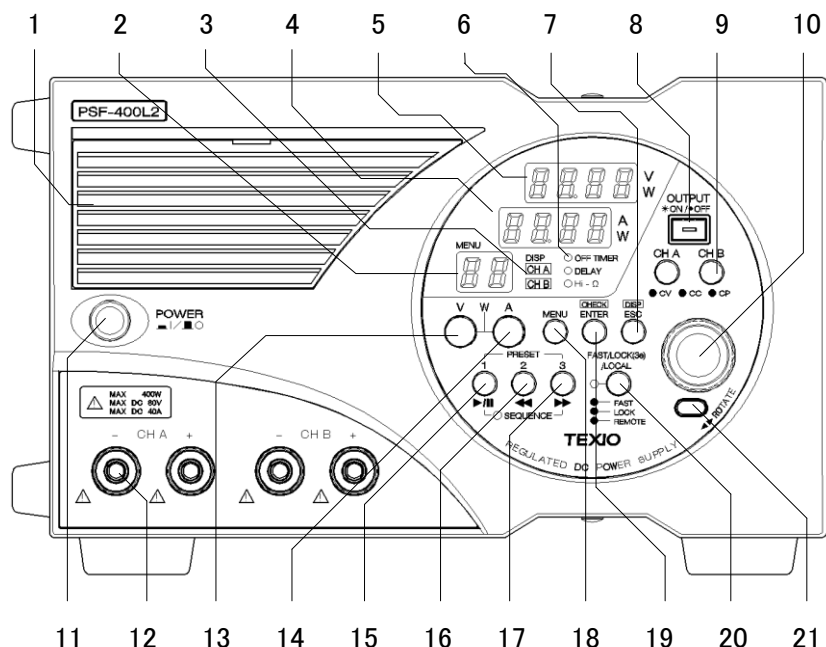
図 4-1 前面図(PSF-400L2)
