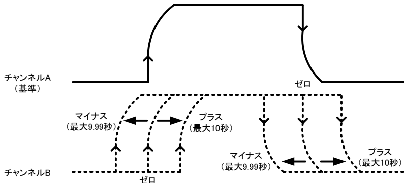
図 5-12 ディレイ機能の時間概念
