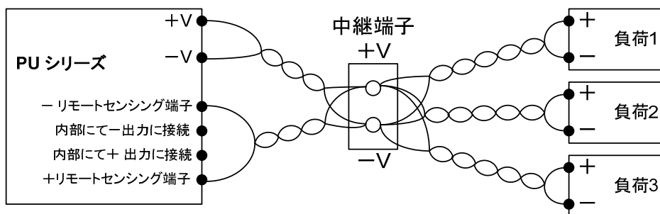
図 2-26 リモートセンシングによる中継端子を用いた複数の負荷への接続
