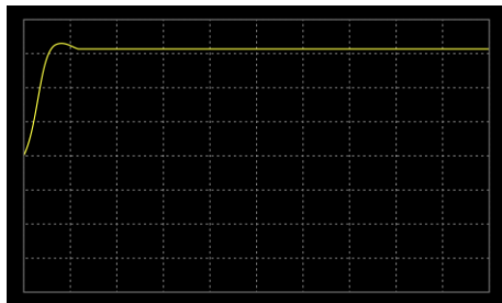
ARB11 2次ステップ応答(減衰係数 0.7)
