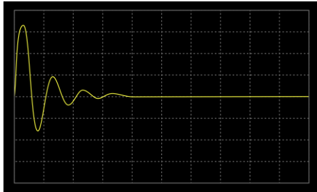
ARB14 2次インパルス応答(減衰係数 0.7)
