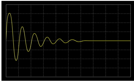
ARB13 2次インパルス応答(減衰係数 0.2)
