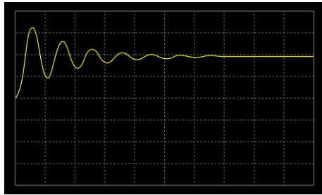
ARB10 2次ステップ応答(減衰係数 0.2)
