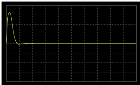
ARB14 2次インパルス応答(減衰係数 0.7)
