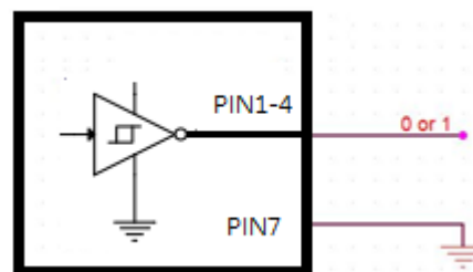
ピン 1-4 出力 配線図
