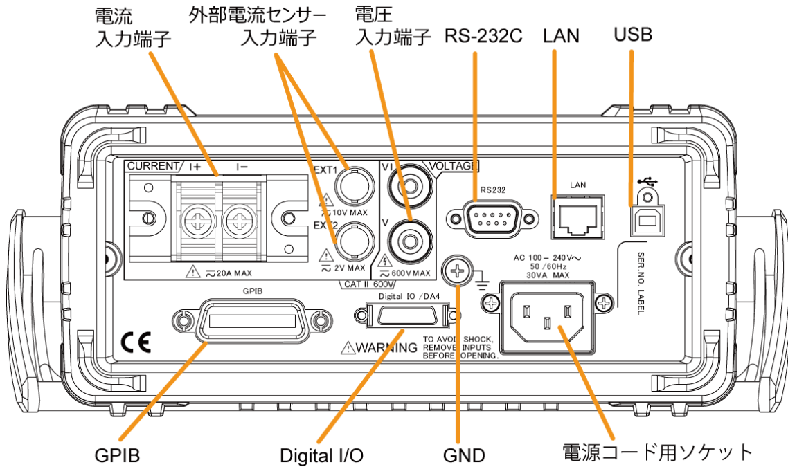
電源コード用ソケット
