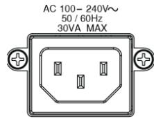
電源コード用ソケット
