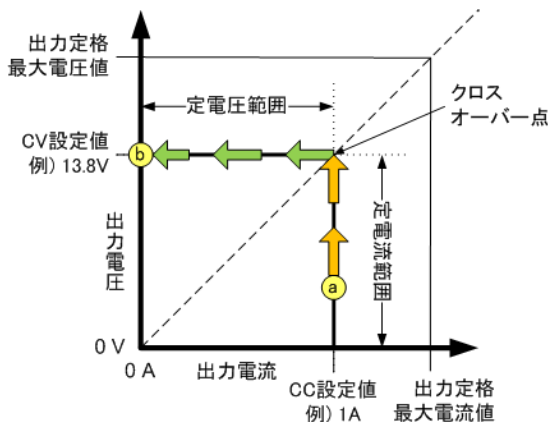
図 5-1 定電圧/定電流特性
