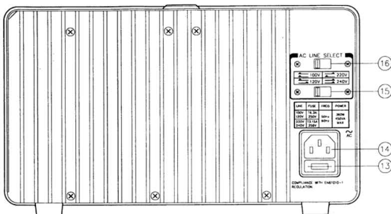
図 4-4 GPR-M リアパネル
