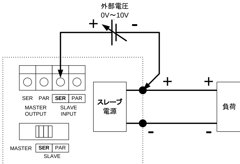
図 5-4 出力電圧制御
