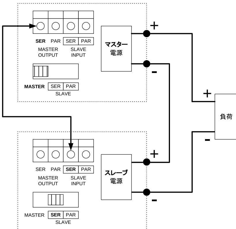
図 5-2 直列接続
