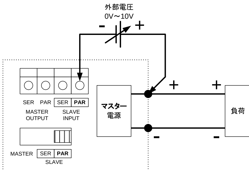
図 5-5 出力電流制御
