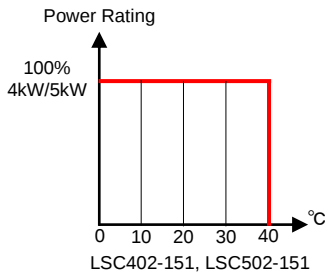
周囲温度に対する電力定格
