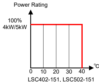
周囲温度に対する電力定格
