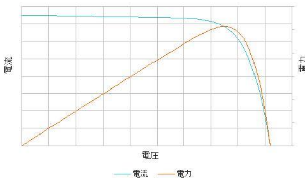
I-V, P-V特性
