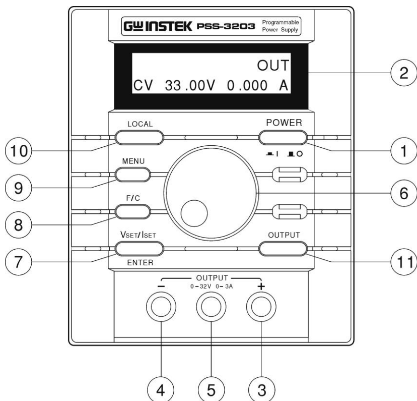
図 4.1 フロントパネル
