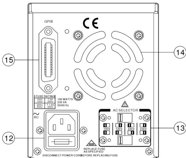
図 4-2 リアパネル
