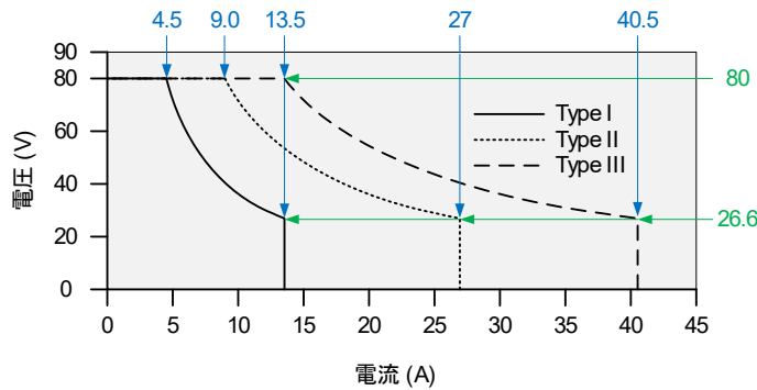
PSW 160V シリーズ 出力範囲
