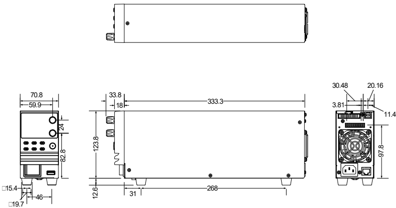
PSW-360M250/PSW-360H800(mm)
