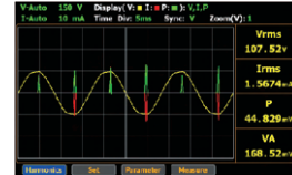
グラフ表示 (ウェーブフォーム)
